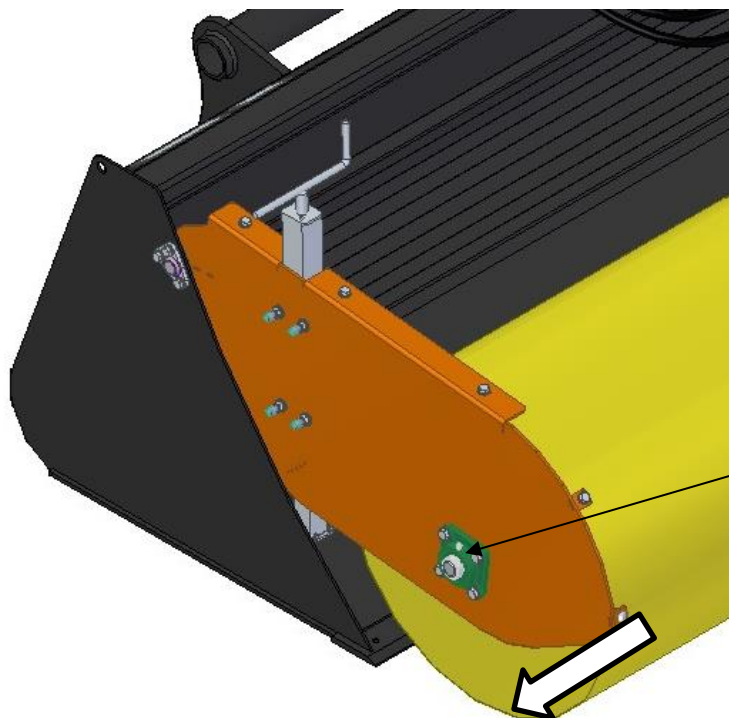
Rysunek 11. Demontaż szczotki.
