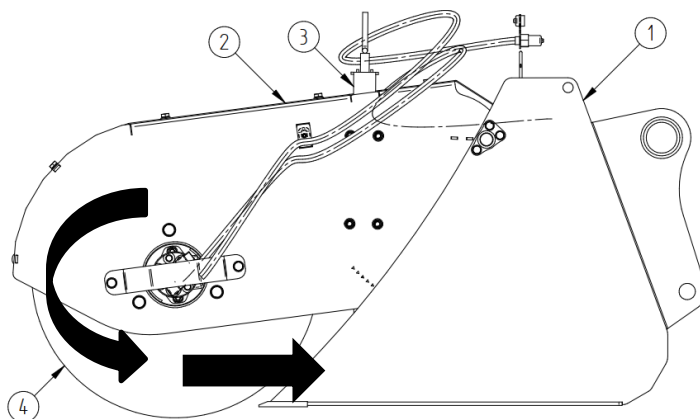
Rysunek 5. Opis zasada działania łyżko-zamiatarki (1) łyżka, (2) pokrywa, (3) stopa podporowa, (4) szczotka,
