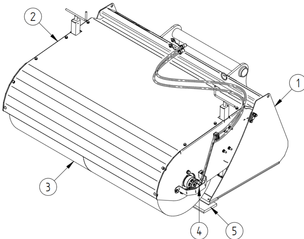
Rysunek 13. Budowa ogólna.
