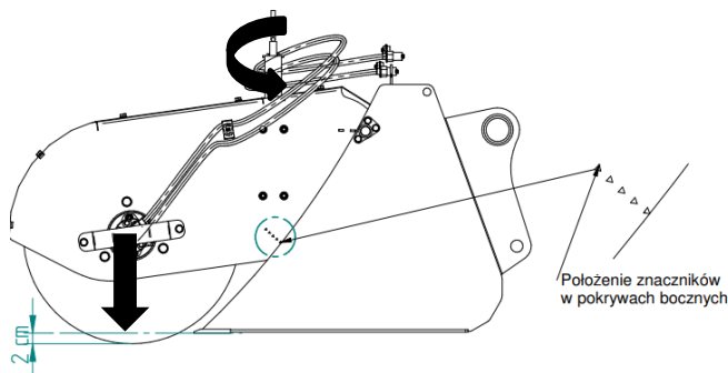
Rysunek 7a. Regulacja docisku szczotki - regulacja szczotki do dołu.
